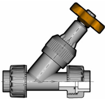
Угловой вентиль VVUIV PBX с разборными муфтовыми окончаниями, EPDM, FIP d25 (DN20)
