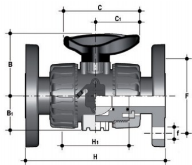
Шаровой кран промышленного применения VKD ХПВХ с фланцевыми окончаниями d50 (DN40)
