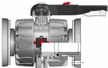
Шаровой кран промышленного применения VKD С фланцевыми окончаниями (уплотнение EPDM) PP-H d90 (DN80)
