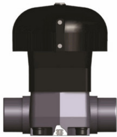
Мембранный клапан DK ПБХ с пневмоприводом, PN10, фланцевые окончания, EPDM, FIP d90 (DN80)
