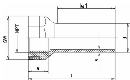
Адаптер переходной с внутренней резьбой ПВДФ (Simona) 20x1/2" SDR21 PN16
