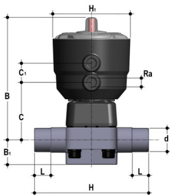
Мембранный клапан DK ХПВХ с пневмоприводом ДвД, PN10, втулочные окончания d40
