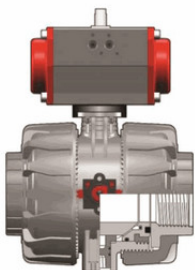
Шаровой кран VKD ПВХ с пневмоприводом НЗ с резьбовыми окончаниями, EPDM, FIP R4" (DN90)
