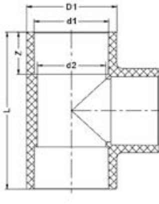
Тройник для раструбной сварки 90° PP-H IPS d40 PN10
