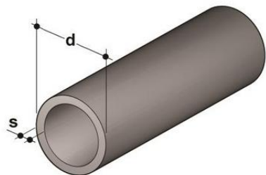
Напорная труба ПВДФ d63 SDR33 PN10
