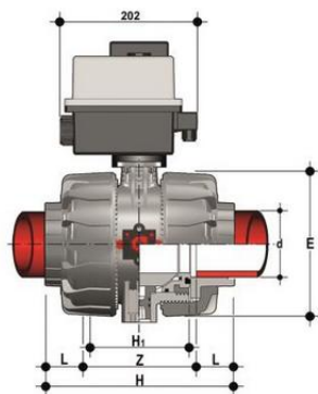
Шаровой кран VKD с эл.приводом 24V AC/DC, муфтовые окончания, DN65-100 (уплотнение EPDM) PP-H d110 (DN100)
