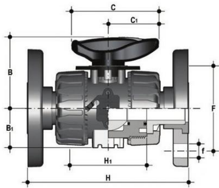
Шаровой кран ПВХ для регулирования потока VKR с фланцевыми окончаниями, FKM, FIP d20 (DN15)
