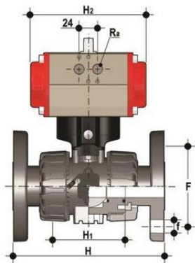
Шаровой кран VKD ПВДФ с пневмоприводом ДвД с фланцевыми окончаниями d50 (DN40)
