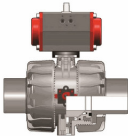
Шаровой кран VKD ПВДФ с пневмоприводом НЗ с резьбовыми окончаниями d90 (DN80)
