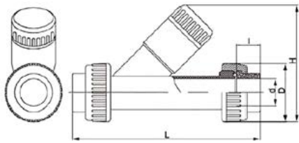
Фильтр сетчатый (грязевой) PP-H IPS d63 (DN50)
