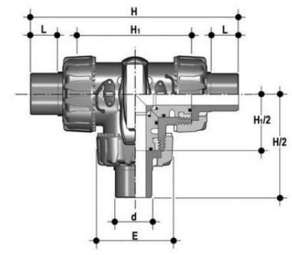
3-х ходовой шаровой кран ТКД с втулочными окончаниями L-шар (уплотнение EPDM) PP-H d40 (DN32)
