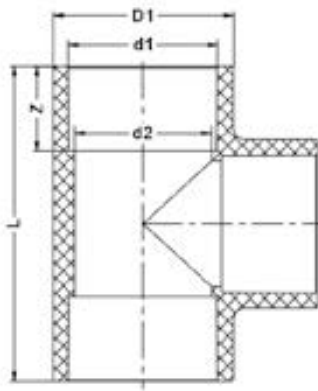
Тройник для раструбной сварки 90° PP-H IPS d63 PN10
