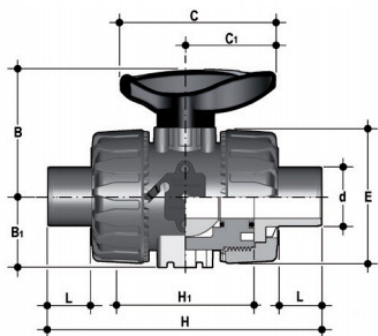
Шаровой кран ПВХ промышленного применения VKD со втулочными окончаниями, FKM, FIP d32 (DN25)
