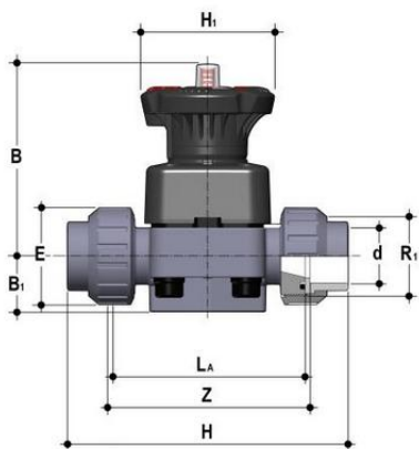
Мембранный клапан DKUIV PBX с разборными муфтовыми окончаниями, FKM, FIP d50 (DN40)
