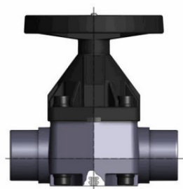
Мембранный клапан VMDV ПВХ с втулочными окончаниями, EPDM, FIP d110 (DN100)
