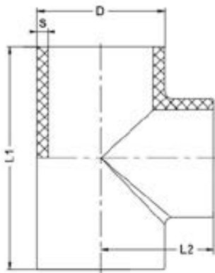
Тройник для стыковой сварки 90° PP-H IPS d20 PN10
