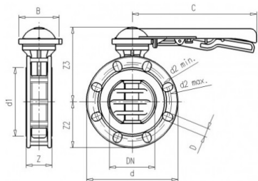
Дисковый затвор ПВХ с рукояткой, EPDM, VDL d90 (DN80)
