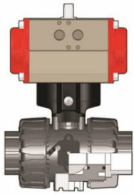
Шаровой кран VKD ХПВХ с пневмоприводом НО с муфтовыми окончаниями; DN65-100 d75 (DN63)
