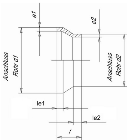
Муфта редукционная PP-H Simona 110x75 SDR11 PN6
