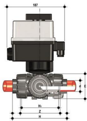
3-х ходовой шаровой кран ТКД с эл.приводом 90-240V, муфтовые окончания, Т-шар (уплотнение FKM) PP-H d40 (DN32)
