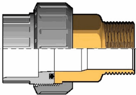
Муфта разборная с НР ПВХ (латунь) FIP 16x3/8
