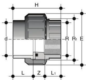
Муфта разборная с ВР ПВХ FIP 25x3/4"
