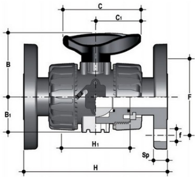
Шаровой кран ПВХ промышленного применения VKD с фланцевыми окочаниями, EPDM, FIP d40 (DN32)
