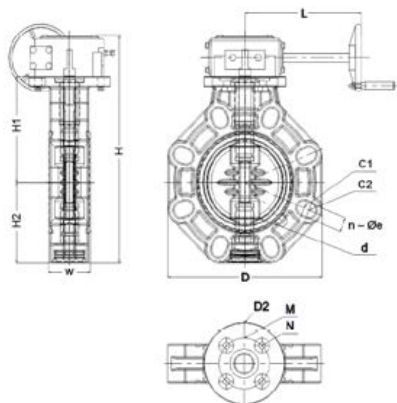
Затвор дисковый ПБХ с редуктором промышленный IPS (Model A) d8" (DN200)
