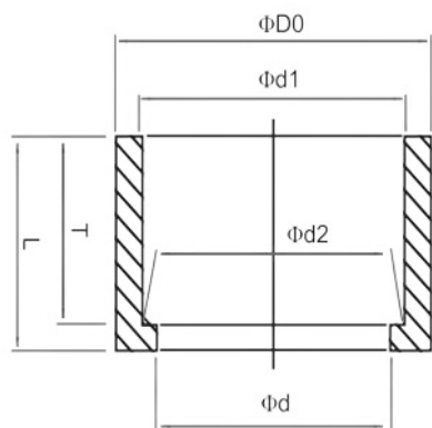
Кольцо переходное ПВХ IPS 63x20
