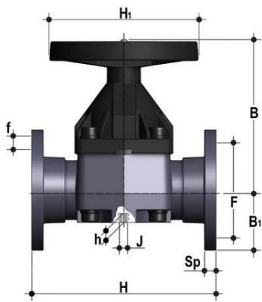
Мембранный клапан VM ПВХ с фланцевыми окончаниями d90 (DN80)
