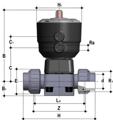
Мембранный клапан ДК ХПВХ с пневмоприводом НО, РН10, разборные муфтовые окончания d63 (DN50)
