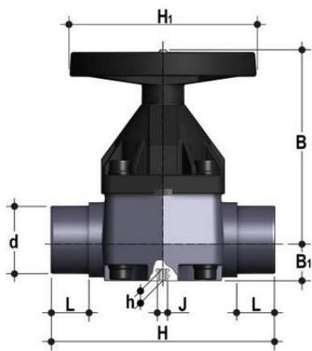
Мембранный клапан VMDM с втулочными окончаниями (уплотнение FKM / мембрана PTFE) PP-H d90 (DN80)
