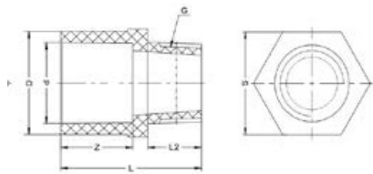
Муфта переходная для раструбной сварки с НР РР-Н IPS d25 PN10
