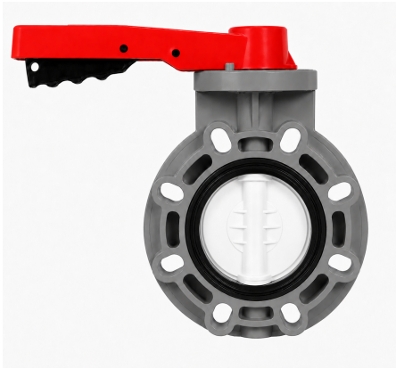
Затвор дисковый в корпусе FRPP (диск - ПВДФ) с рукояткой промышленного применения EPDM IPS d140 (DN125)
