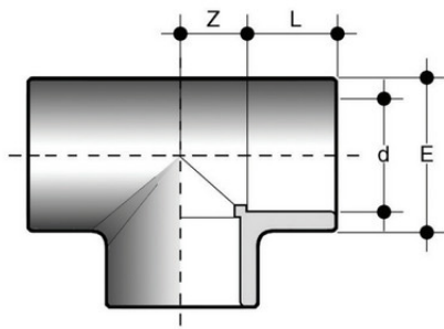
Тройник равнопроходной клеевой 90° ПВХ IPS d315
