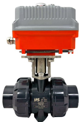
Шаровой кран IVKD ПВХ с эл.приводом (площадка IPQ) 220V, муфтовые окончания, EPDM, IPS d25 (DN20)
