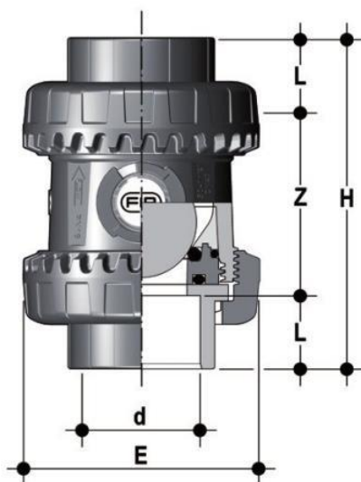
Шаровой обратный клапан SXEIV PBX; с муфтовыми окончаниям, EPDM, FIP d50 (DN40)
