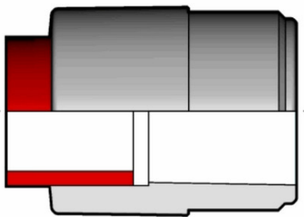
Муфта редукционная для раструбной сварки PP-H FIP 110x90 PN10
