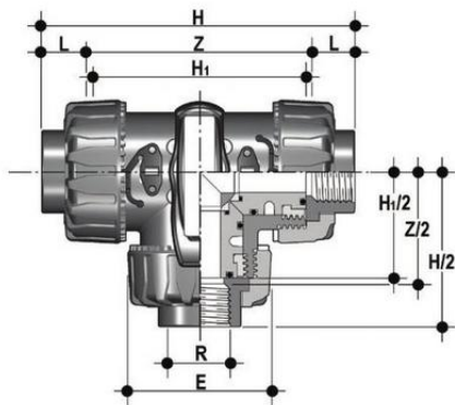
3-х ходовой шаровой кран ТКД ХПВХ с резьбовыми окончаниями, L-шар R1" (DN25)
