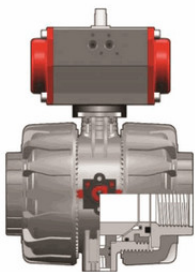
Шаровой кран VKD ПВХ с пневмоприводом НЗ с резьбовыми окончаниями, EPDM, FIP R3" (DN80)
