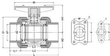
Кран шаровой промышленного применения с муфтовыми окончаниями PP-H IPS d50
