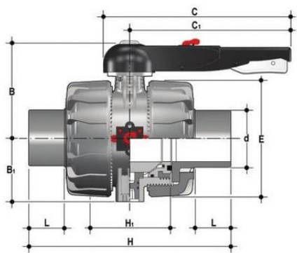
Шаровой кран промышленного применения VKD C втулочными окончаниями (уплотнение EPDM) PP-H d90
