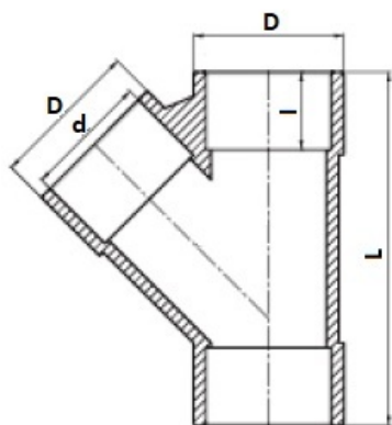
Тройник равнопроходной клеевой 45° ПВХ IPS d75
