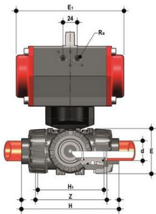
3-х ходовой шаровой кран ТКД с пневмоприводом ДвД с муфтовыми окончаниями, Т-шар (уплотнение EPDM) PP-H d40 (DN32)
