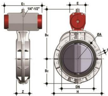
Дисковый затвор FK с пневмоприводом HO (уплотнение EPDM) PP-H d400 (DN400)
