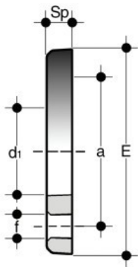
Свободный фланец ПВХ FIP d32
