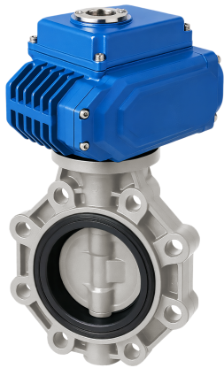
Дисковый затвор IFK PP-H с электрическим приводом 24V DC, FKM, IPS d160 (DN150)
