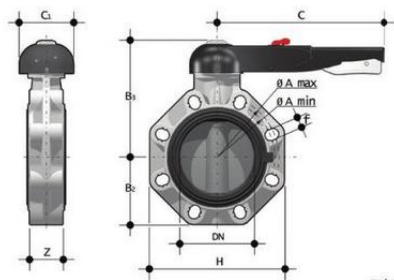
Дисковый затвор ПВХ FKOVLM с рукояткой, FKM, FIP d90 (DN80)
