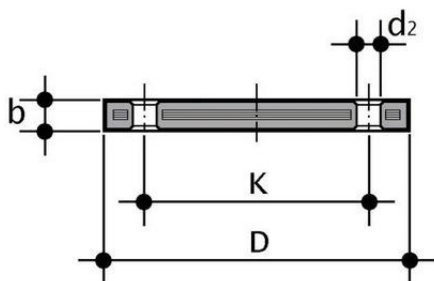
Глухой фланец PP-H FIP d400 PN10
