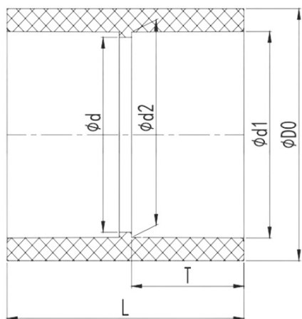
Муфта соединительная ПВХ IPS d40
